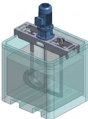
DISEÑO UNIVERSAL TIPO PUENTE CON PALA HELICOIDAL
